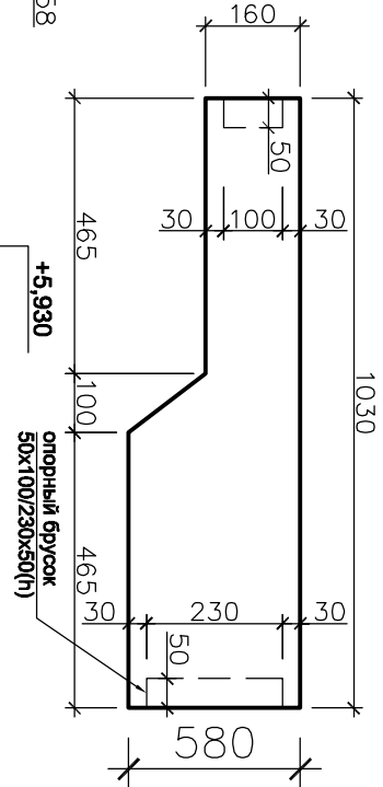
Ступень в плане М 1 : 10
